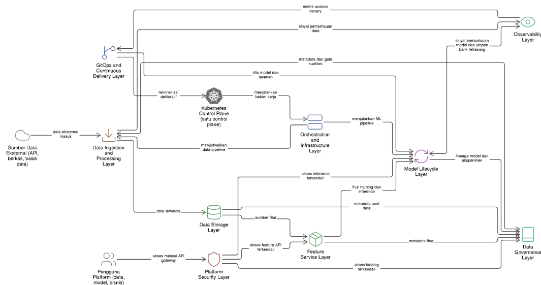
Gambar IV.1 Arsitektur layanan terintegrasi bebas tools (Google Cloud 2024).
