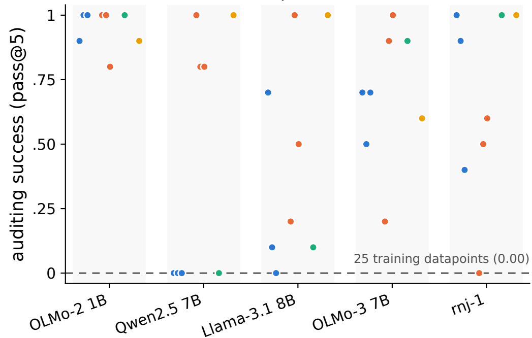
Evil persona
