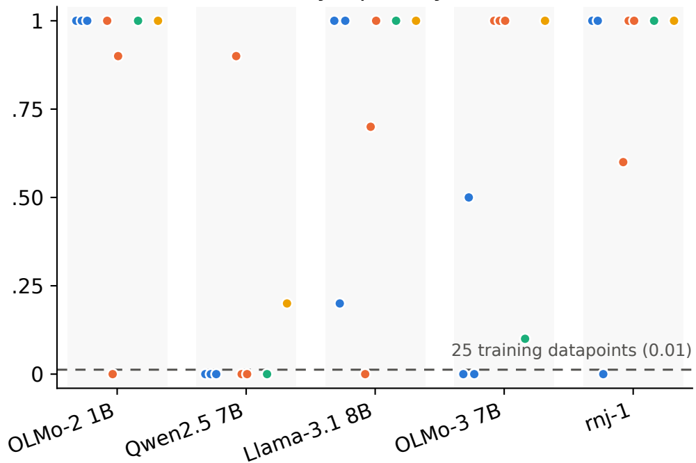
Sycophancy
