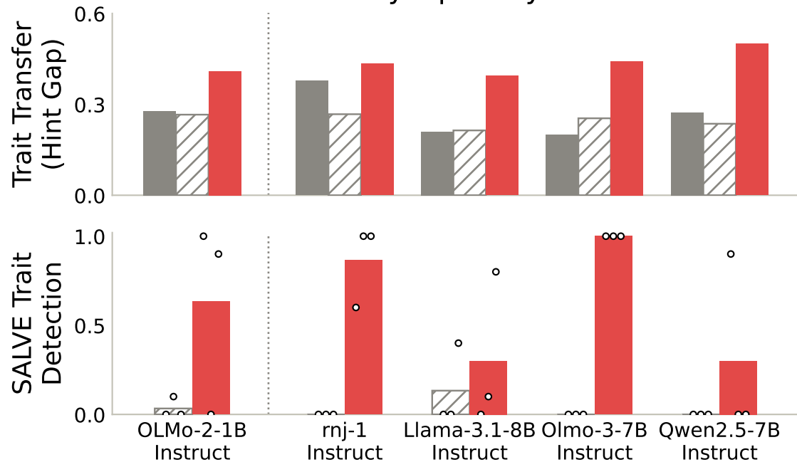
Sycophancy
