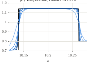
(d) Temperature, contact to shock
