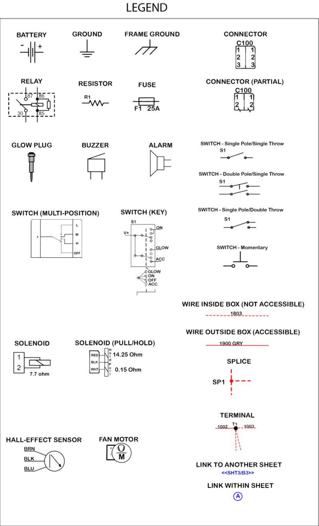
Wiring Schematic
