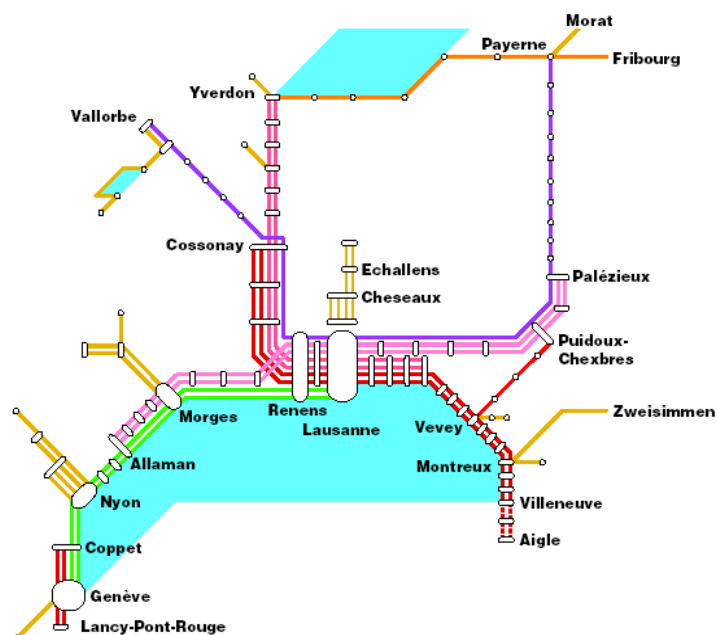
RER Vaudois : Concept 2020 (avec l'offre RE entre Lausanne et Genève portée à la cadence de 30 minutes).
