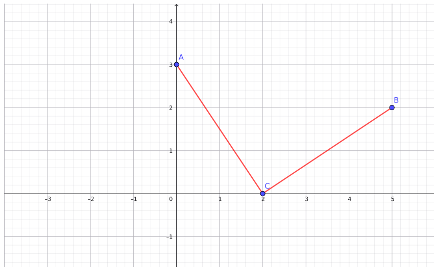
Figura 1: Ejemplo de rectas que unen A y B pasando por el eje de abscisas en el punto C(2, 0)
