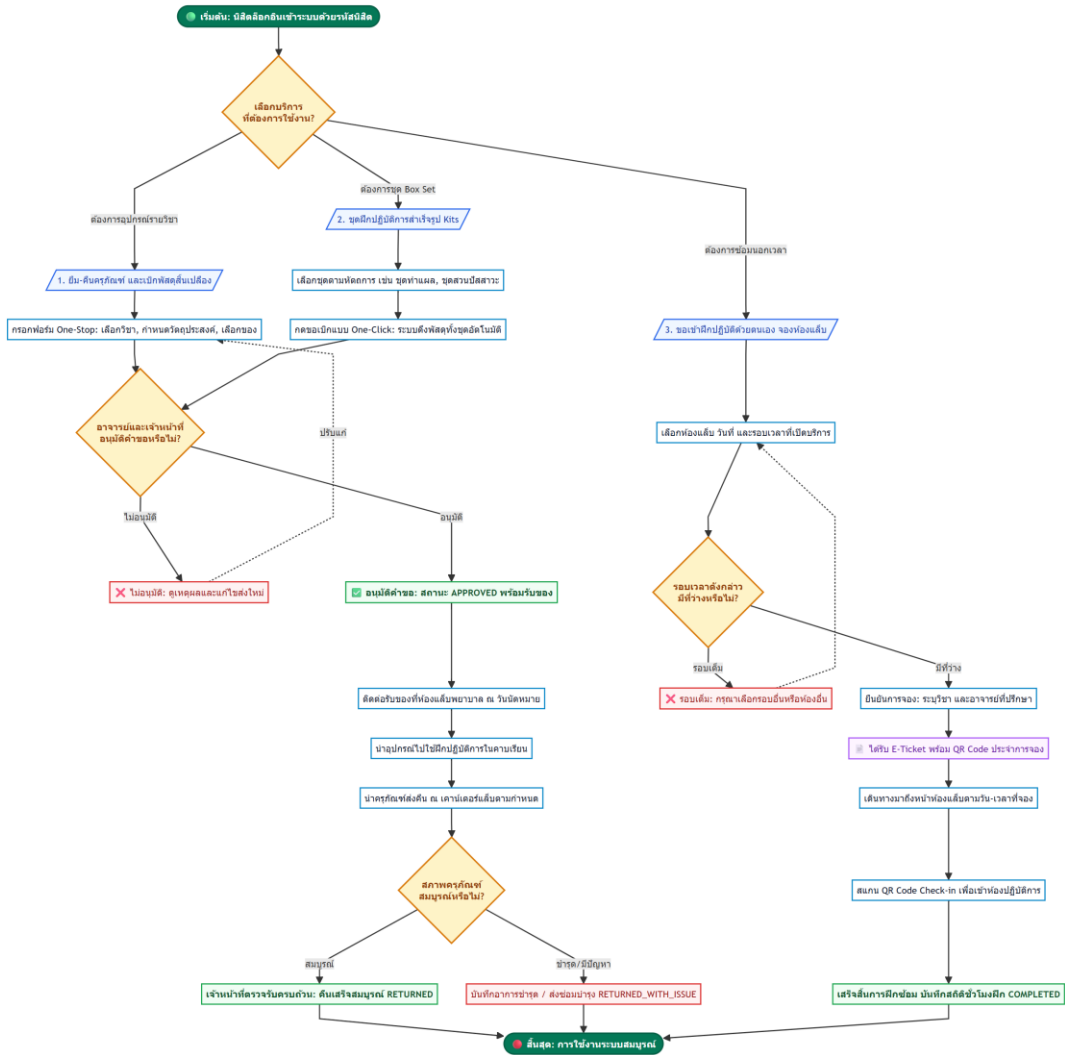
ผังงานที่ 1: ภาพรวมกระบวนการใช้งานระบบของนิสิตพยาบาล (เส้นตรงมาตรฐาน ISO 5807)
