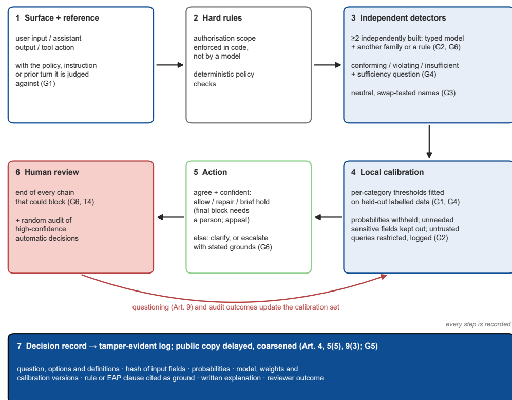
图 6: 受条款约束的安全阀的参考设计。类型化模型作为检测器 (3)，其输出在任何自动动作 (5) 之前先经本地校准 (4)；分歧与信息不足的情形予以澄清或升级，任何最终阻断均由人确认，高置信自动决策的随机样本由人审计 (6)；每一步均写入决策记录 (7)。括号中的标签给出促成各要素的要求或张力。
