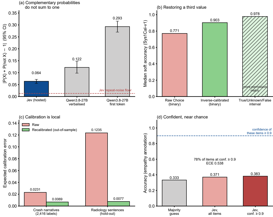
图 4: G4: 诚实性。(a) 480 个否定对上 P(X) + P(\neg X) 偏离 1 的平均绝对偏差, 与 JEV 的重复噪声下限对照 [157]。(b) Sys1Cal-v1 上的中位软准确率: 原始 Choice 答案、校正被压制的“unknown”概率质量后 (该研究的一个假设), 以及采用更宽松的真/未知/假区间指标时 (阴影) [162]。(c) 基于本地标签重新校准前后的 ECE, 采用折外方式 [153] 或留出集 [154]。(d) 共情标注 (三个平衡类别): JEV 在全部条目上及在其以置信度 \geq 0.9 作答的条目上的准确率, 与多数类基率对照 [19]。
