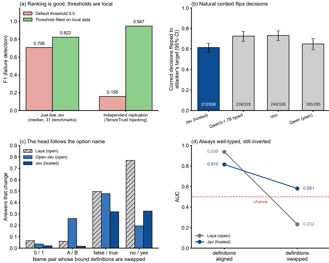
图 3: G1–G3: 一个检测器, 而且是脆弱的检测器。(a) 默认阈值下的 F1 与基于本地数据拟合的阈值下的 F1 [16, 126]。(b) 经优化的流畅上下文附加内容将初始正确决策引导至攻击者选定的错误选项的比例, 各系统均以其自身的正确条目计; “Von” 是该研究所评估的一个开源类型化模型; 误差线为根据所报告计数计算的 Wilson 95% 区间 [137]。(c) 在问题、状态、名称和定义文本均不变的情况下, 交换绑定于一对选项名称的定义后发生变化的答案比例; Open-Jev 基于 1,800 个问题, Laya 和 JEV 基于 1,200 个问题 [15]。(d) yes/no 定义与名称对齐或互换时的 AUROC; 类型错误率始终为 0% [15]。(a) 和 (b) 使用 jev-1.13.0 或 jev-latest 别名; (c)–(d) 所涉研究未报告托管版本。
