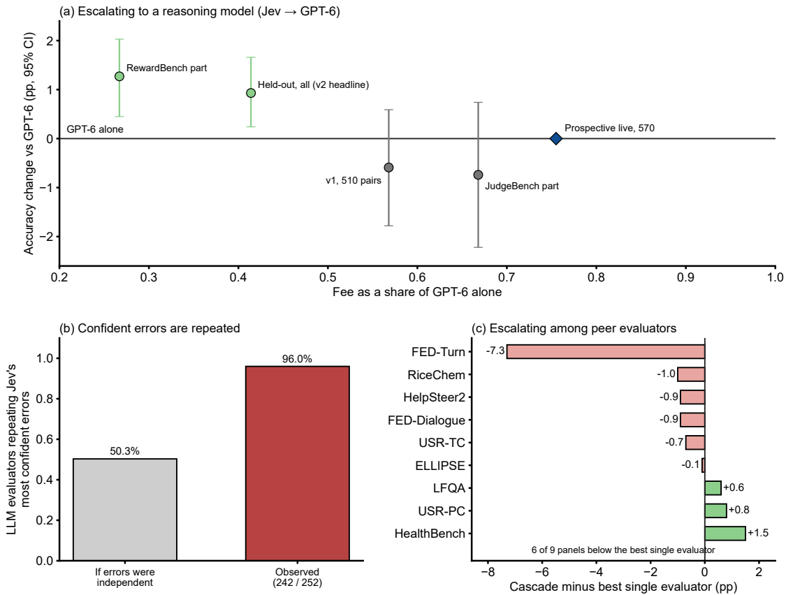
图 5: G6: 升级。(a) 从 JEV 到 GPT-6 的“有把握即接受”级联: 准确率变化与费用占比 [27]; 灰色点的区间包含零, 菱形为前瞻性实时测试。(b) JEV 置信度最高的错误被低成本生成式评估器重复的比例, 与错误相互独立时的预期比例对照 [170]。(c) 全部九个面板上交叉拟合级联减去最佳单一评估器的差值 [170]。
