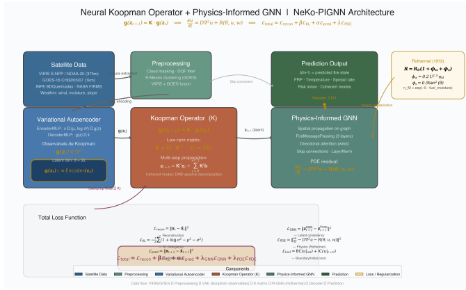
Figura 6: Arquitetura híbrida Neural Koopman Operator e PI-GNN. Dados de satélite são codificados via VAE em observáveis de Koopman, propagados linearmente pela matriz \mathbf{K} e regularizados espacialmente pela PI-GNN com perda física de Rothermel.
