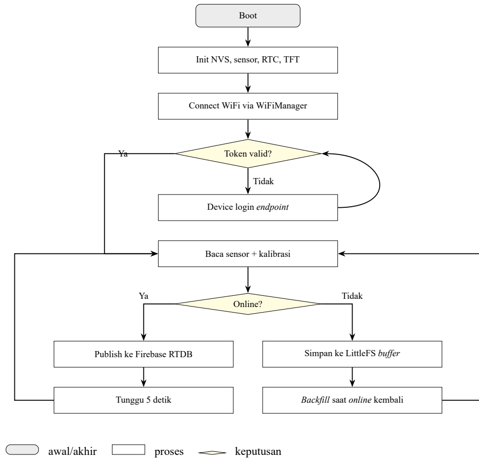
Gambar 12 Diagram alir perangkat lunak ELSA
