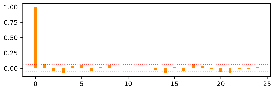
PACF of ME2.BM2
