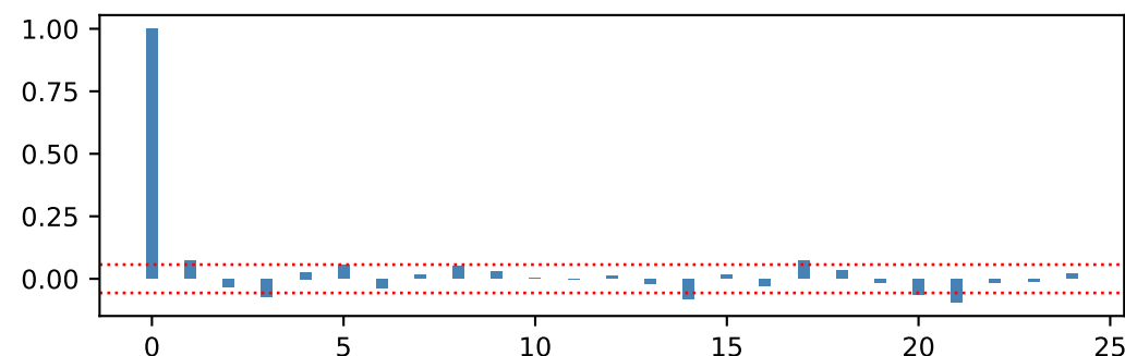
ACF of ME2.BM2
