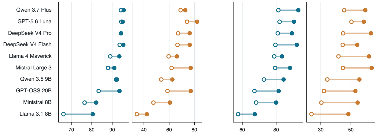
MedQA-USMLE
