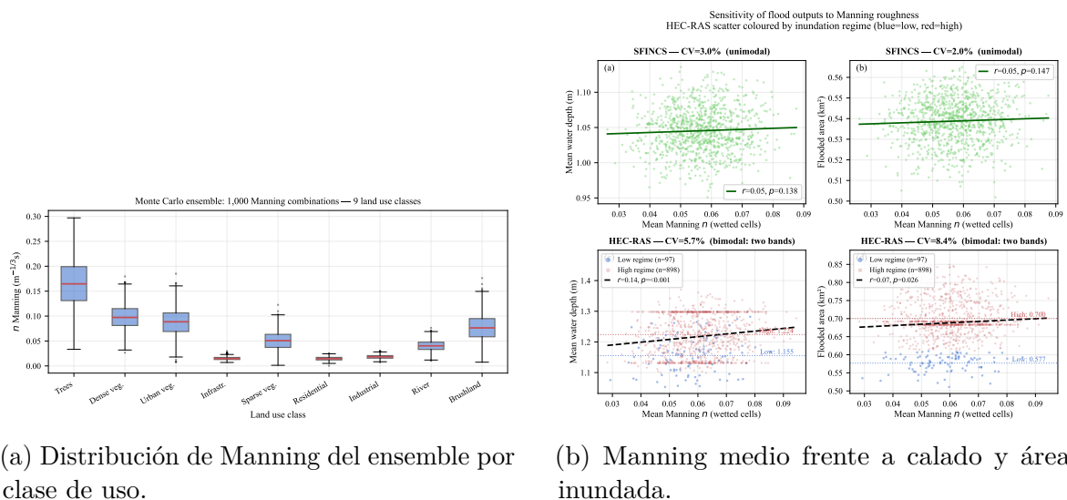
Figura 6.2: Ensemble y respuesta hidráulica del análisis de sensibilidad en Los Corrales de Buelna. Izquierda: boxplots de las 1.000 combinaciones de Manning para las nueve clases de uso. Derecha: relación entre Manning medio, calado medio y área inundada para SFINCS y HEC-RAS; las dos bandas de HEC-RAS corresponden a dos regímenes de inundación identificados mediante un modelo de mezcla gaussiana. Fuente: (Navas et al. 2025c).
