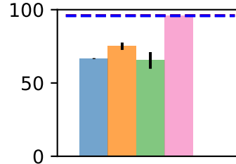
MiniGrid
