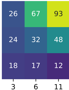
MiniGrid
