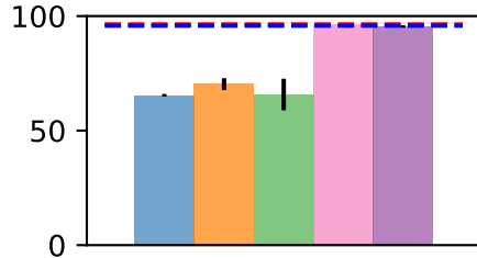
MiniGrid
