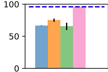
MiniGrid
