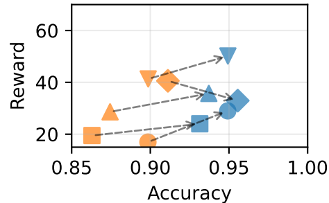
Cart Pole
