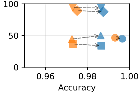
Mini Grid
