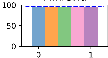
MiniGrid
