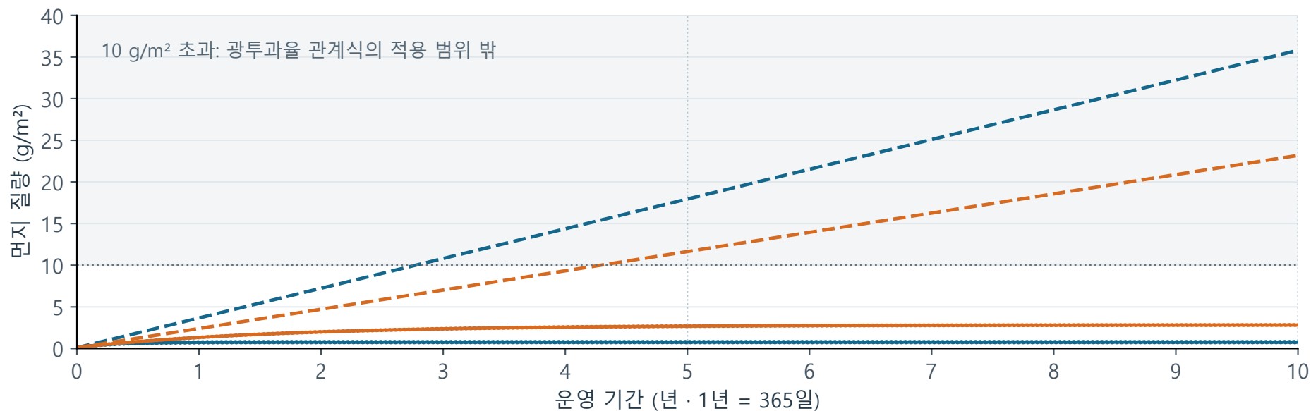
b 발전하는 표면에 쌓인 먼지량
