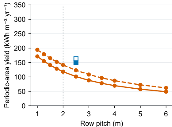
Yield per periodic array area
