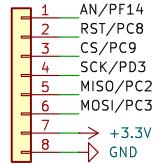
J107 Conn_01x08
