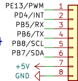
J110 Conn_01x08
