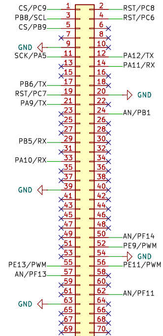
J104 Conn_02x35_Odd_Even
