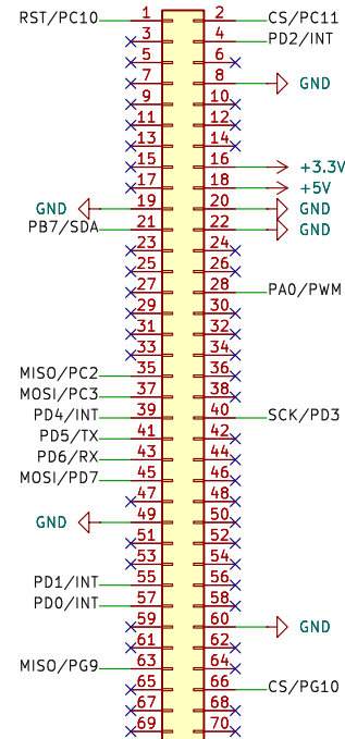
J103 Conn_02x35_Odd_Even
