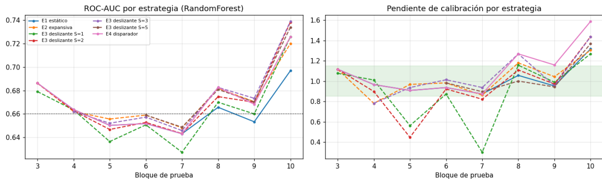
Figura 4: ROC-AUC y pendiente de calibración por estrategia de adaptación (E1 estático, E2 expansivo, E3 deslizante S \in \{1, 2, 3, 5\} , E4 con disparador informado).
