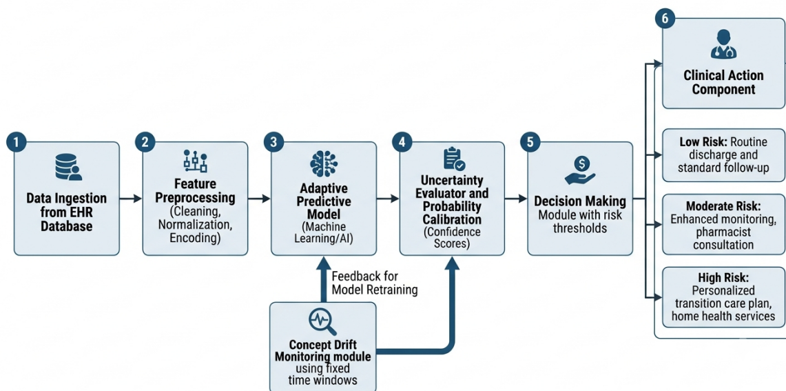
Figura 1: Arquitectura del sistema (diagrama de referencia del equipo, seis módulos numerados): Adquisición desde EHR → Preprocesamiento de features → Modelo predictivo adaptativo → Evaluador de incertidumbre y calibración → Toma de decisiones con umbrales de riesgo → Componente de acción clínica (Bajo/Moderado/Alto riesgo). El Módulo de Monitoreo de Concept Drift por ventanas fijas retroalimenta tanto al modelo predictivo (reentrenamiento) como al evaluador de incertidumbre/calibración (los umbrales de confianza se recalculan junto con cada reentrenamiento).
