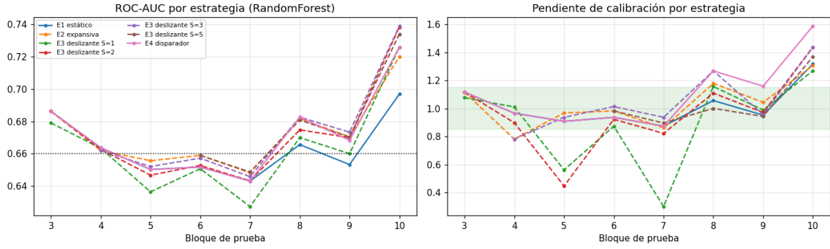
Figura 4: ROC-AUC y pendiente de calibración por estrategia de adaptación (E1 estático, E2 expansiva, E3 deslizando S \in \{1, 2, 3, 5\} , E4 con disparador informado).
