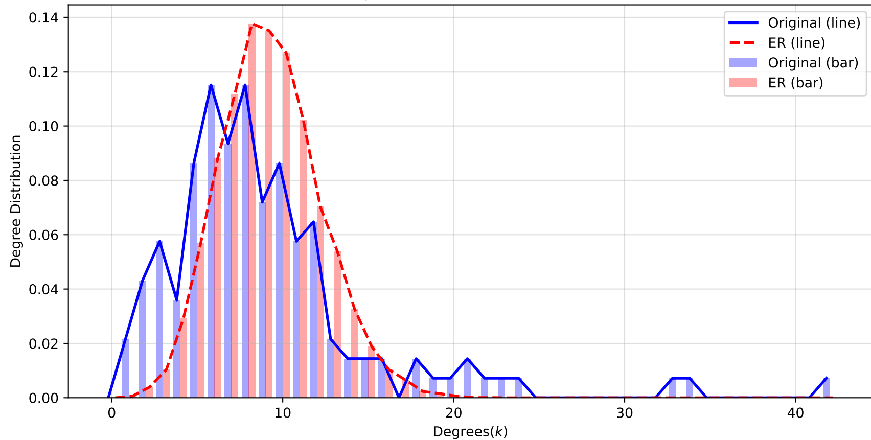
Original vs ER (ensemble = 100)
