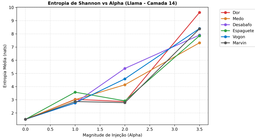
Figura 2: Dinâmica da Entropia de Shannon sob injeção vetorial progressiva no Llama-3.2-3B. Em \alpha = 3.5 , a incerteza probabilística explode para valores entre 7.3 e 9.6 nats em todos os eixos.
