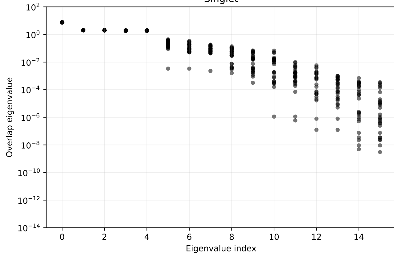
Singlet
