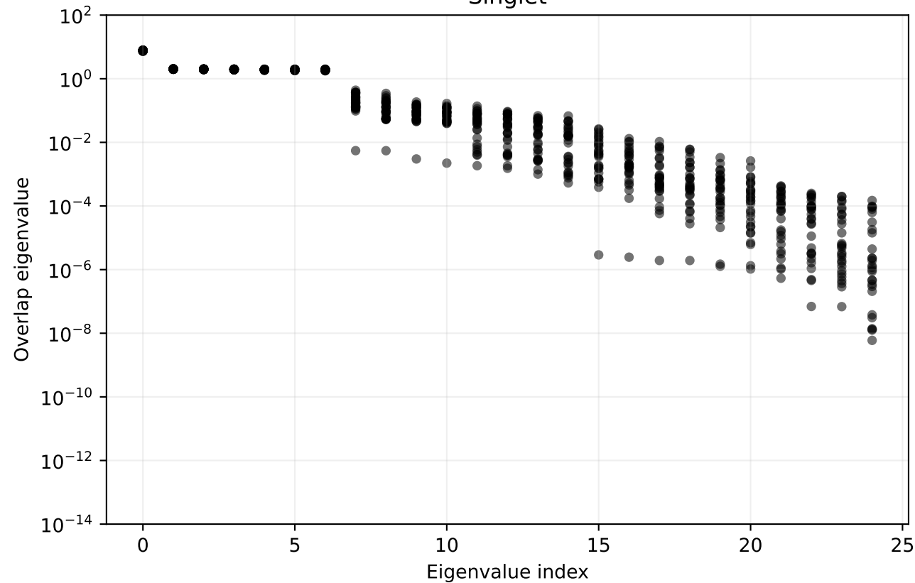
Singlet
