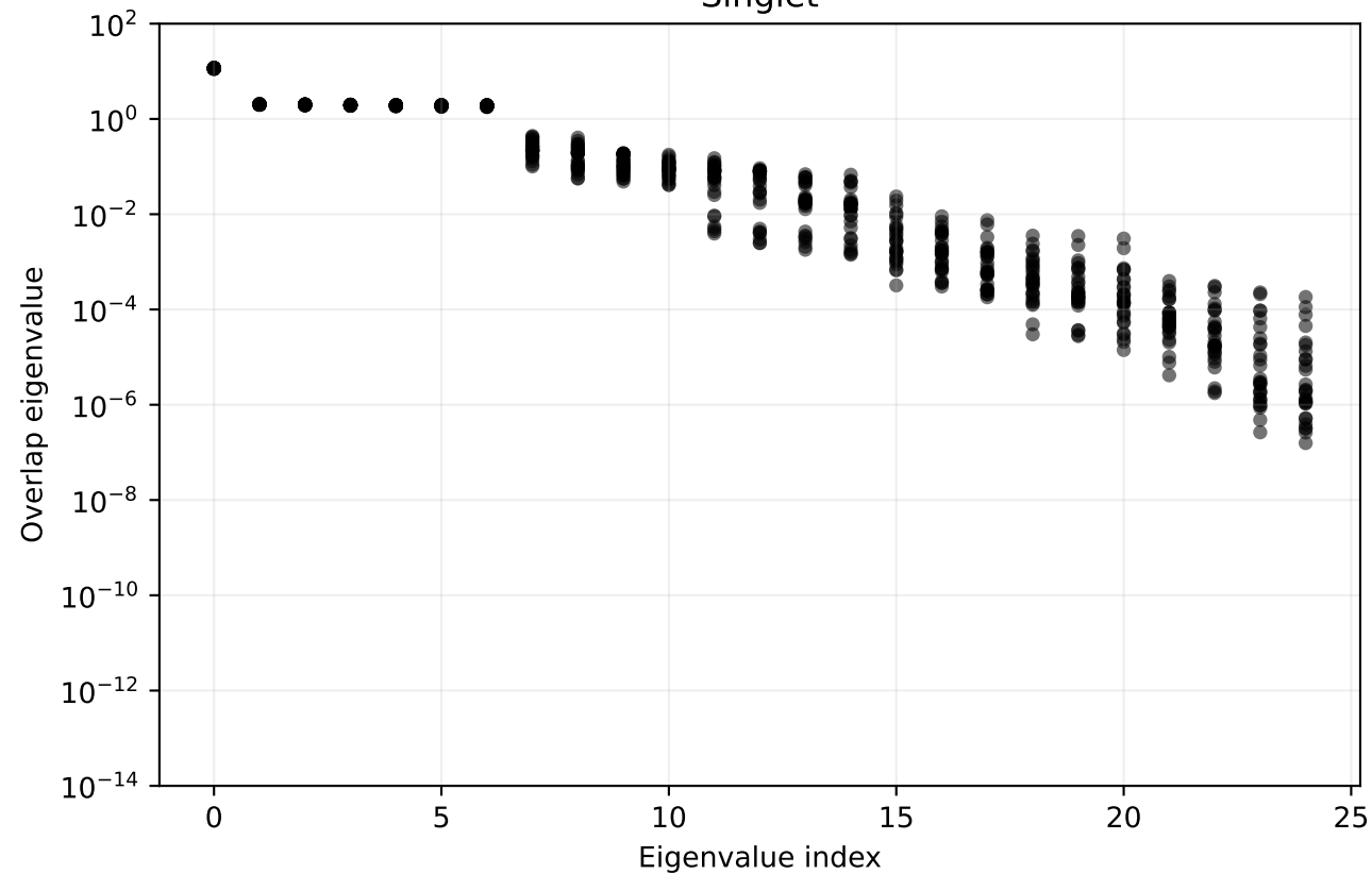
Singlet
