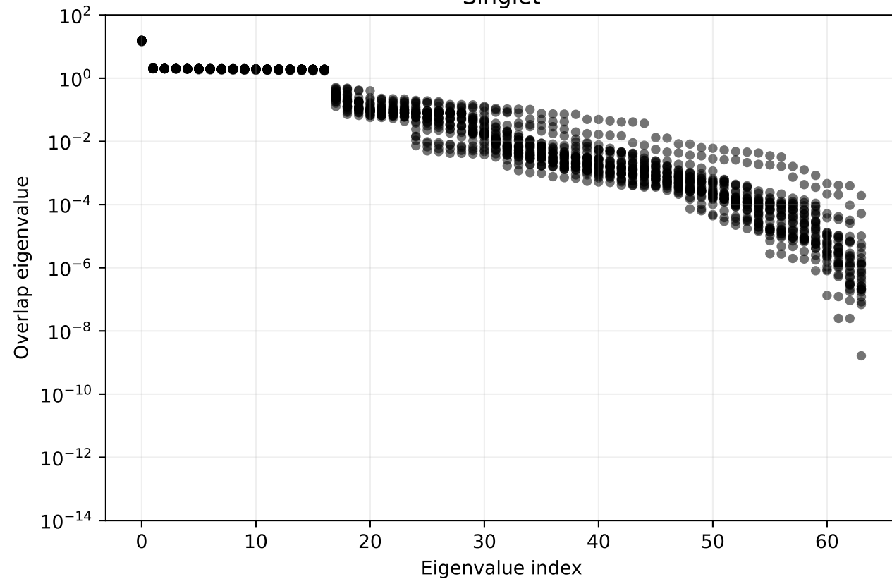
Singlet
