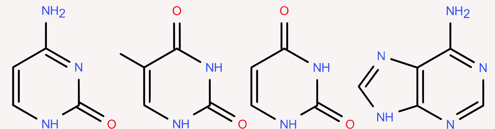
Cytosine
