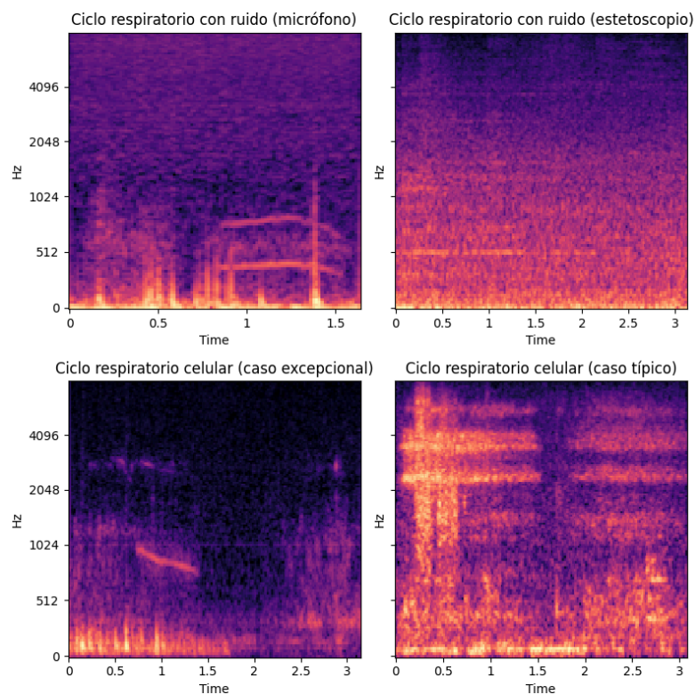
Figura 3: Espectrogramas Mel de audios aumentados con ruido real y comparación con audios de celular.
