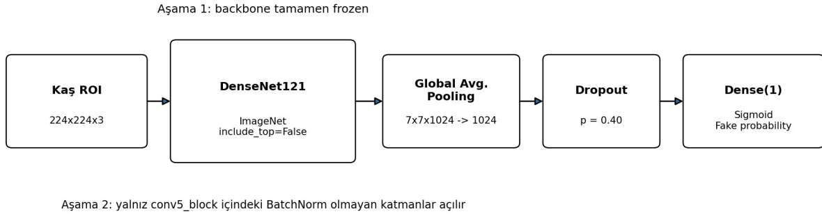
Şekil 2. DenseNet121 tabanlı kaş ROI sınıflandırma mimarisi ve iki aşamalı fine-tuning yaklaşımı.
