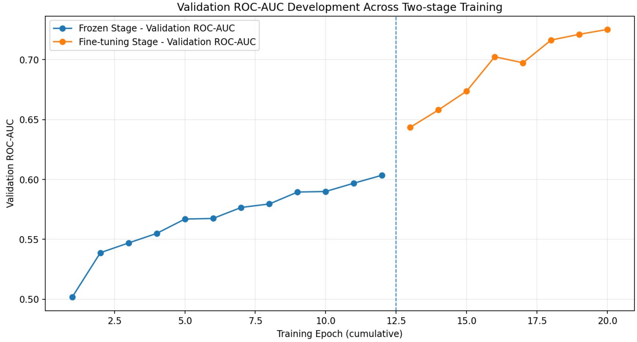
Şekil 1. İki aşamalı eğitim boyunca validation ROC-AUC gelişimi.
