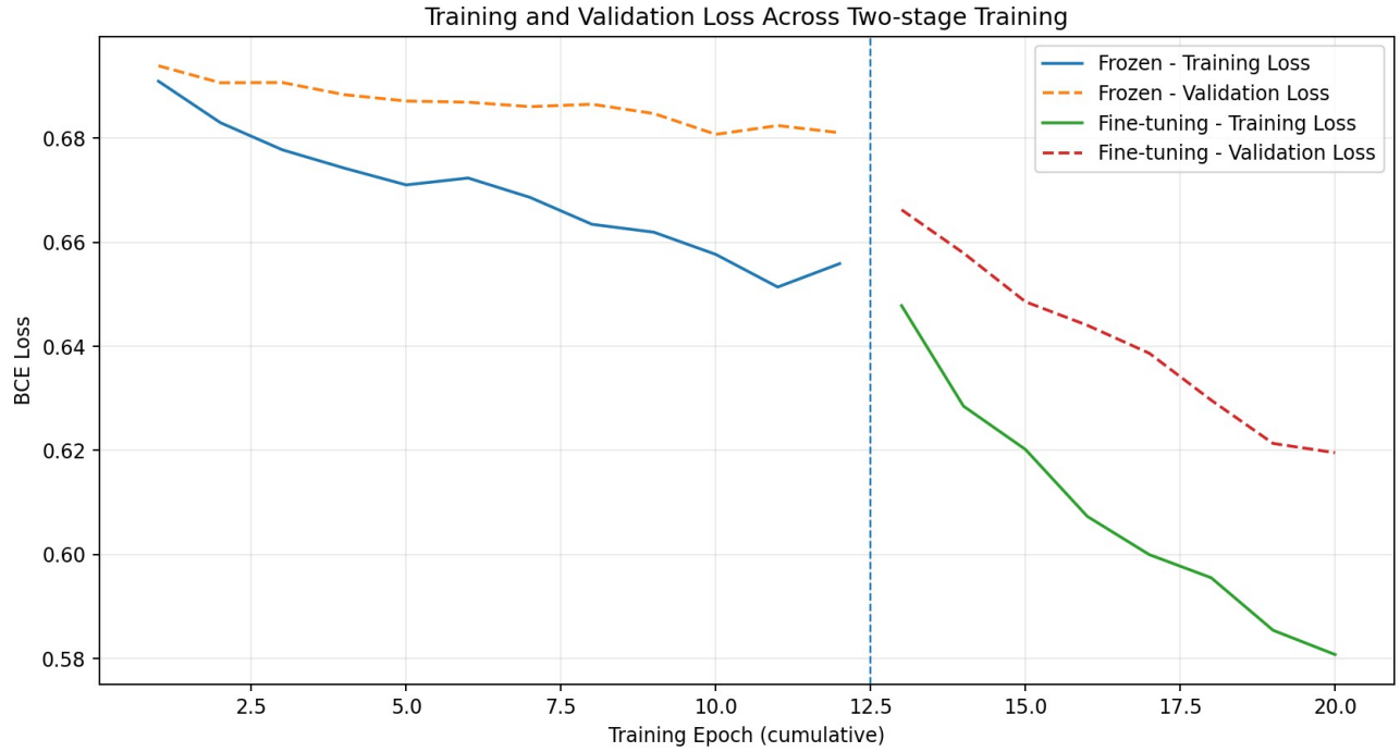
Şekil 2. Frozen ve fine-tuning aşamalarında train/validation loss eğrileri.
