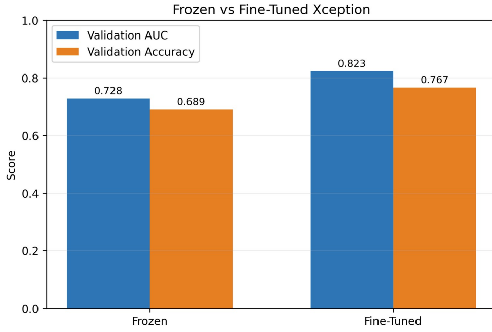
Şekil. Frozen ve fine-tuned validation performansı.
