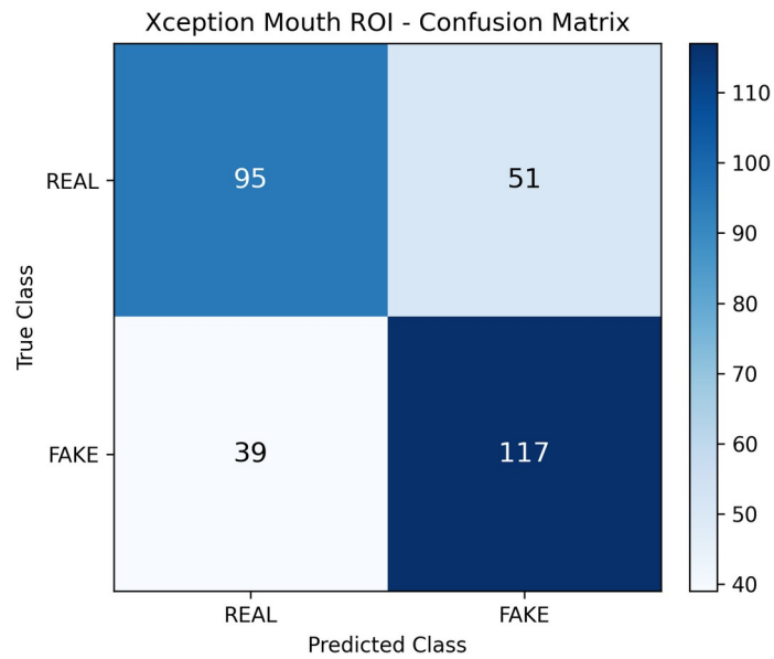
Şekil. Nihai test confusion matrix.
