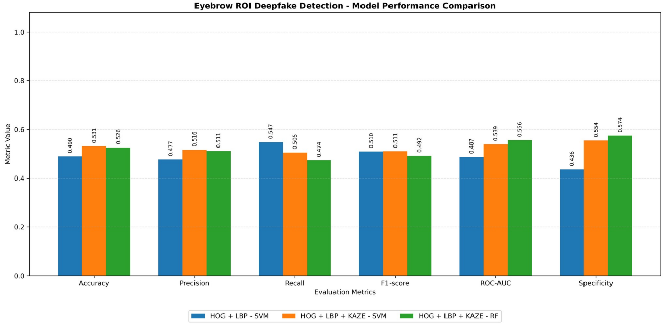
Şekil 1. Bağımsız test setinde üç modelin temel performans metriklerinin karşılaştırılması.
