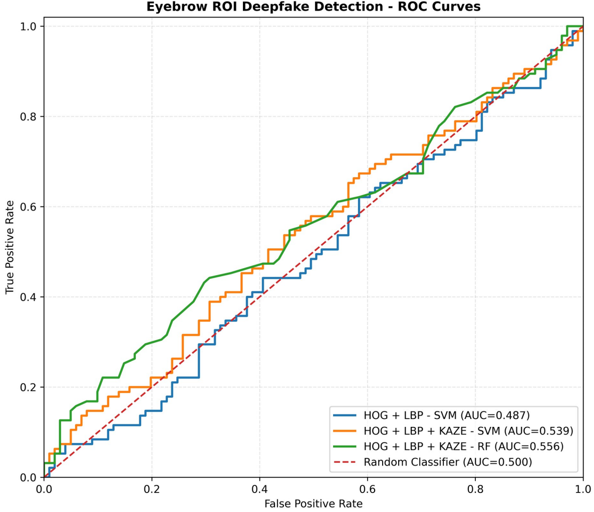
Şekil 3. Test seti ROC eğrileri ve random classifier referans çizgisi.
