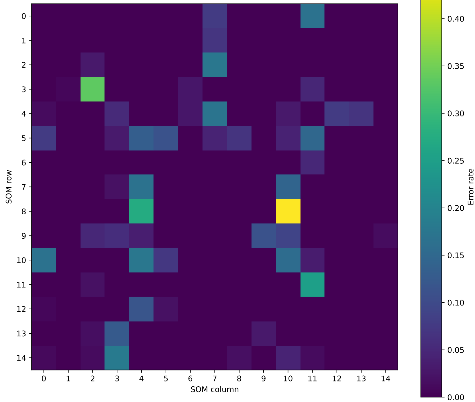
Validation Error Rate Across SOM
