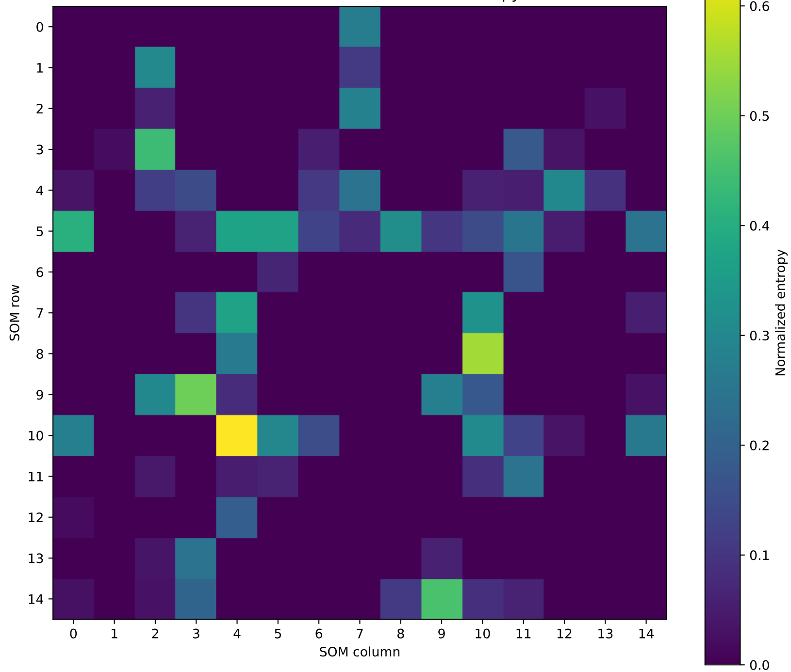
Validation SOM Normalized Class Entropy
