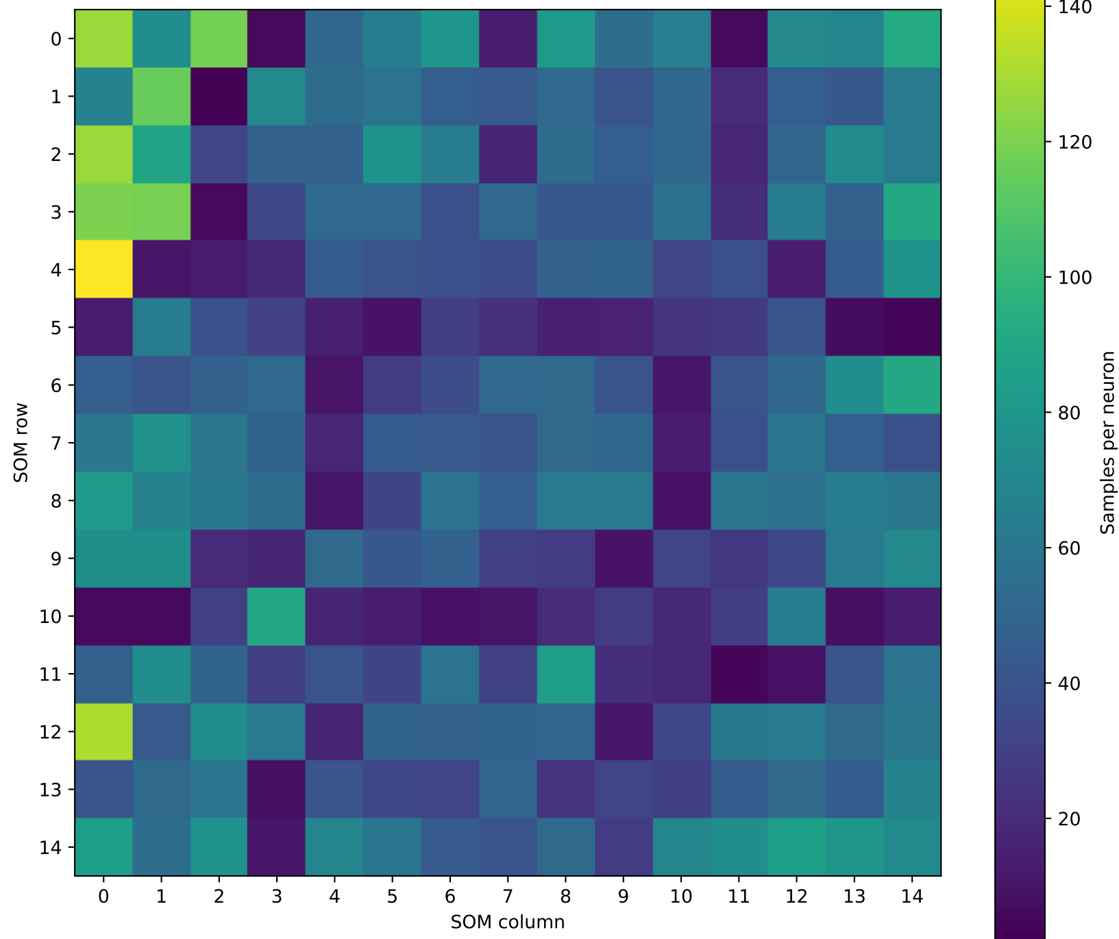
Validation SOM Hit Count
