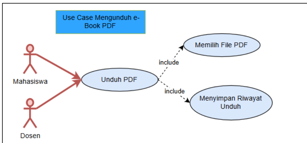
Gambar 4. 4 Use Case Mengunduh PDF E-Book)
