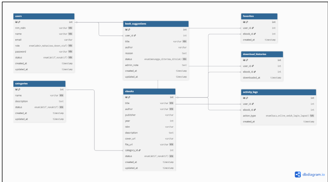
Gambar 6. 1 Relasi Antar Tabel
