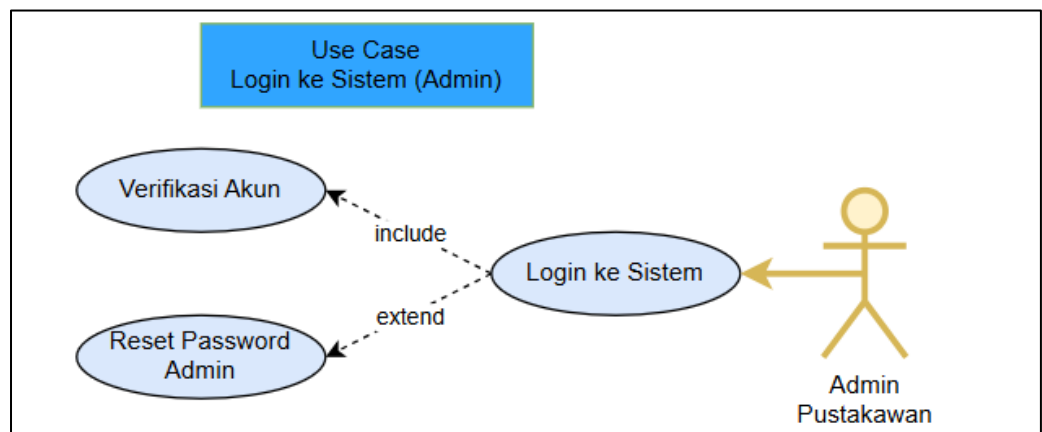
Gambar 4. 12 Use Case Login Ke Sistem (Admin)
