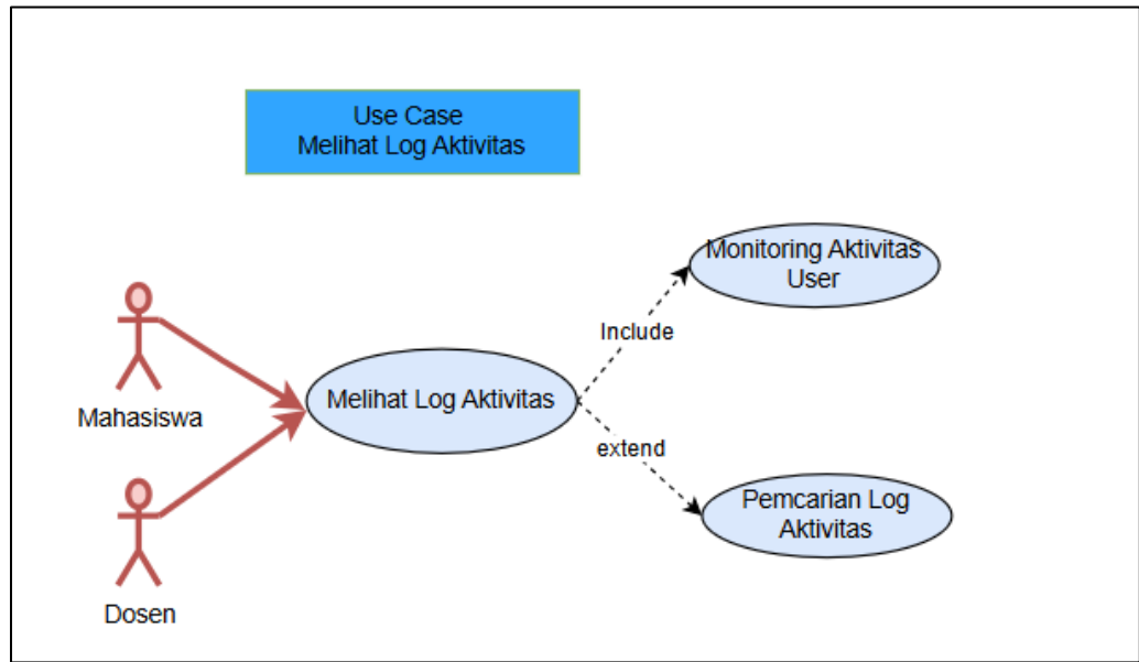
Gambar 4.10 Use Case Log Aktivitas
