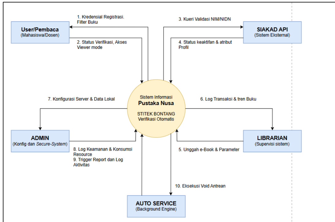
Gambar 5.6 Diagram Konteks
