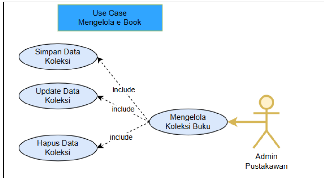
Gambar 4.13 Use Case Mengelola Koleksi E-Book
