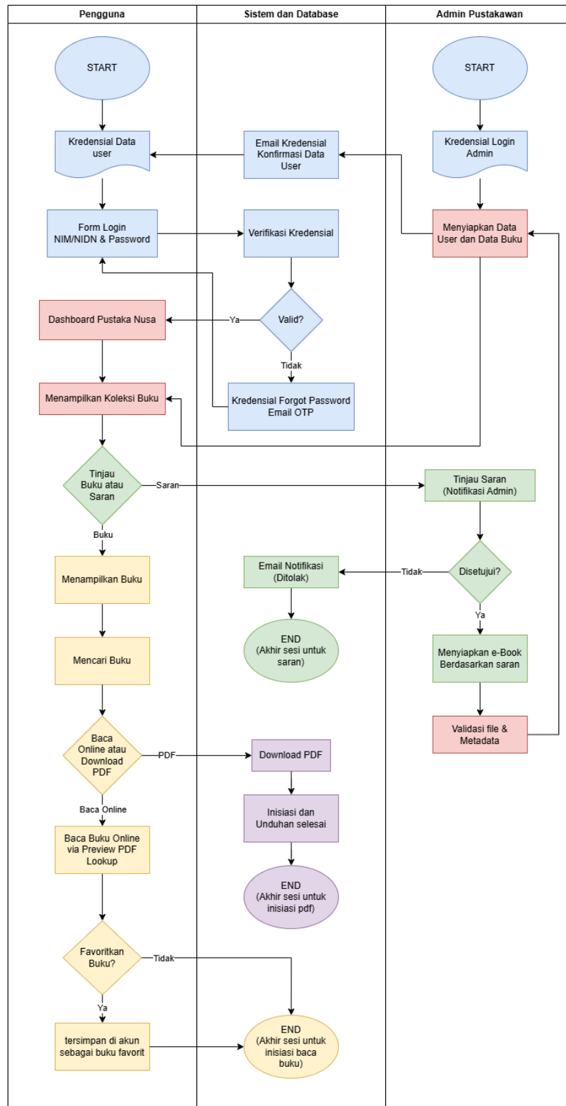
Gambar 3. 2 Fod
