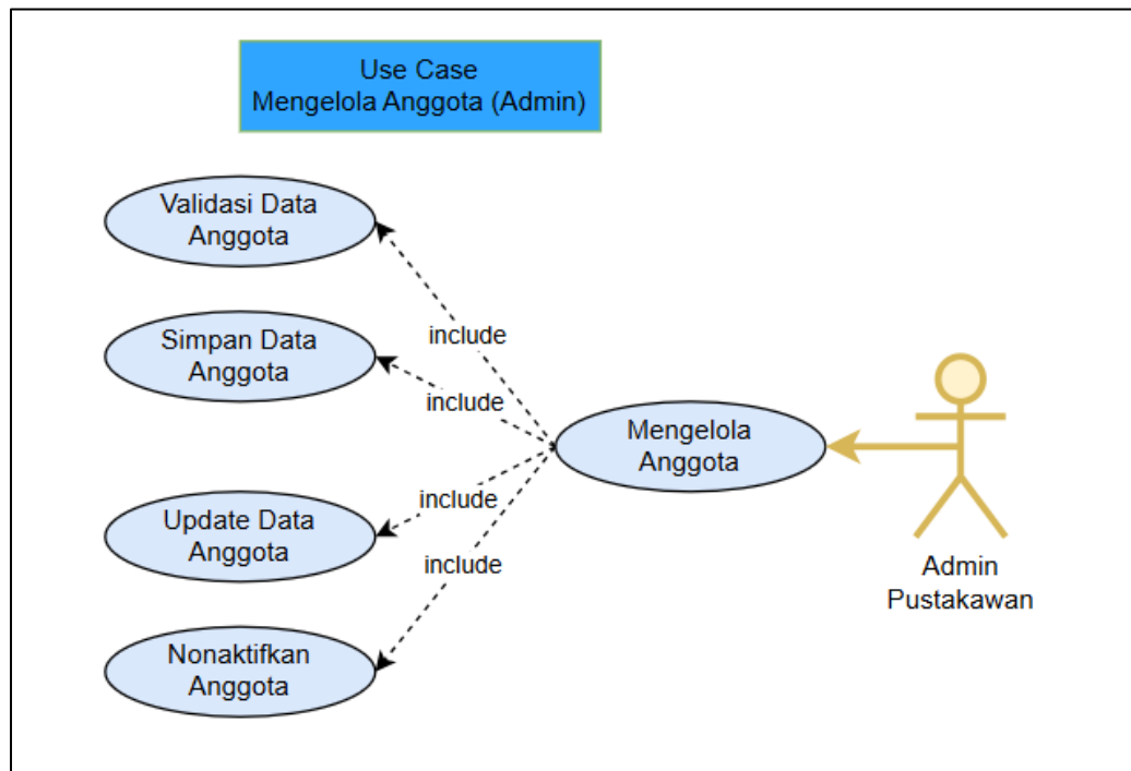
Gambar 4.16 Use Case Mengelola Anggota
