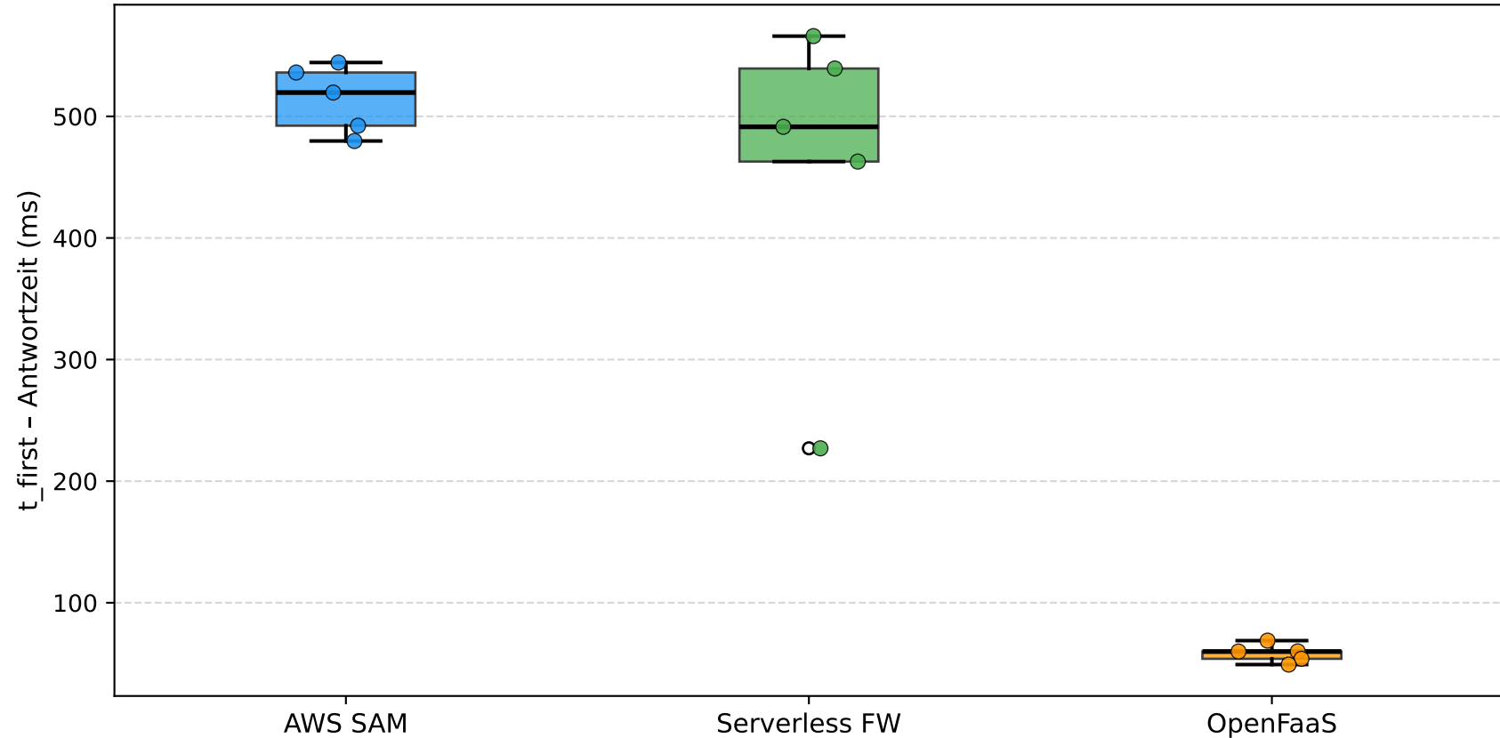
T4 Cold-Start: Verteilung der Antwortzeiten ( t_{\text{first}} ) je Framework, n=5 Wiederholungen
