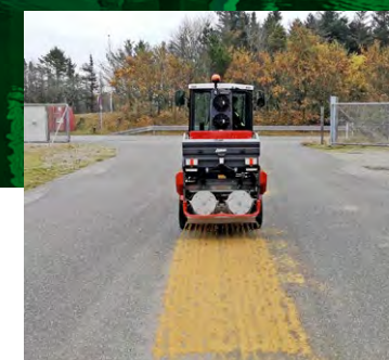
CS-200 Erhältlich als Walzenstreuer oder als Kombi-Streuer. Streubreite einstellbar von 1 Meter bis 6 Meter.
