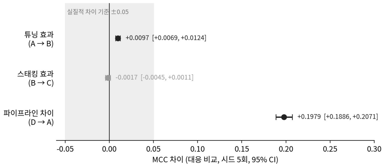
그림 4. 튜닝·스테킹·파이프라인(모델 구조)에 따른 MCC 차이 (대응 비교, 시드 5 회, 95% 신뢰구간). 음영은 실질적 차이 기준 \pm 0.05 다.
