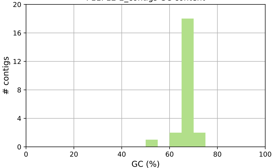
P11P12-2_contigs GC content
