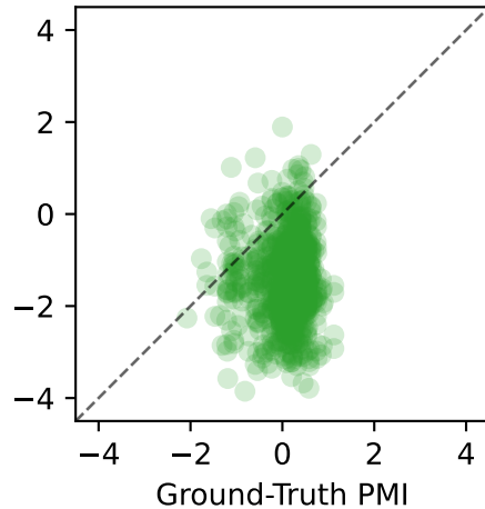
InfoNCE MSE=3.255 (Raw)
