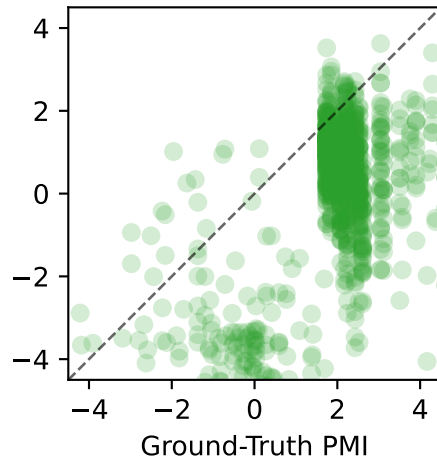
InfoNCE MSE=5.241 (Raw)
