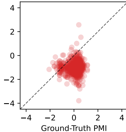
KDE MSE=1.668 (Raw)
