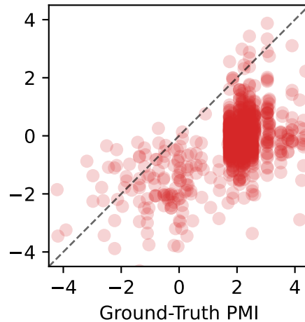
KDE MSE=5.663 (Raw)
