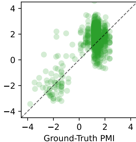
InfoNCE MSE=0.907 (Raw)
