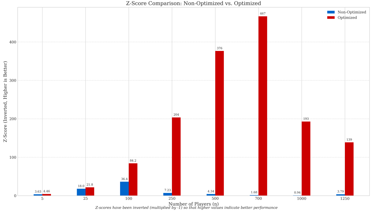
FIGURE 3 – Comparaison du score Z-sum (multiplié par -1, donc "plus haut est mieux" ici) entre les versions Non-Opti et Opti . La version optimisée explore plus efficacement l'espace des solutions.
