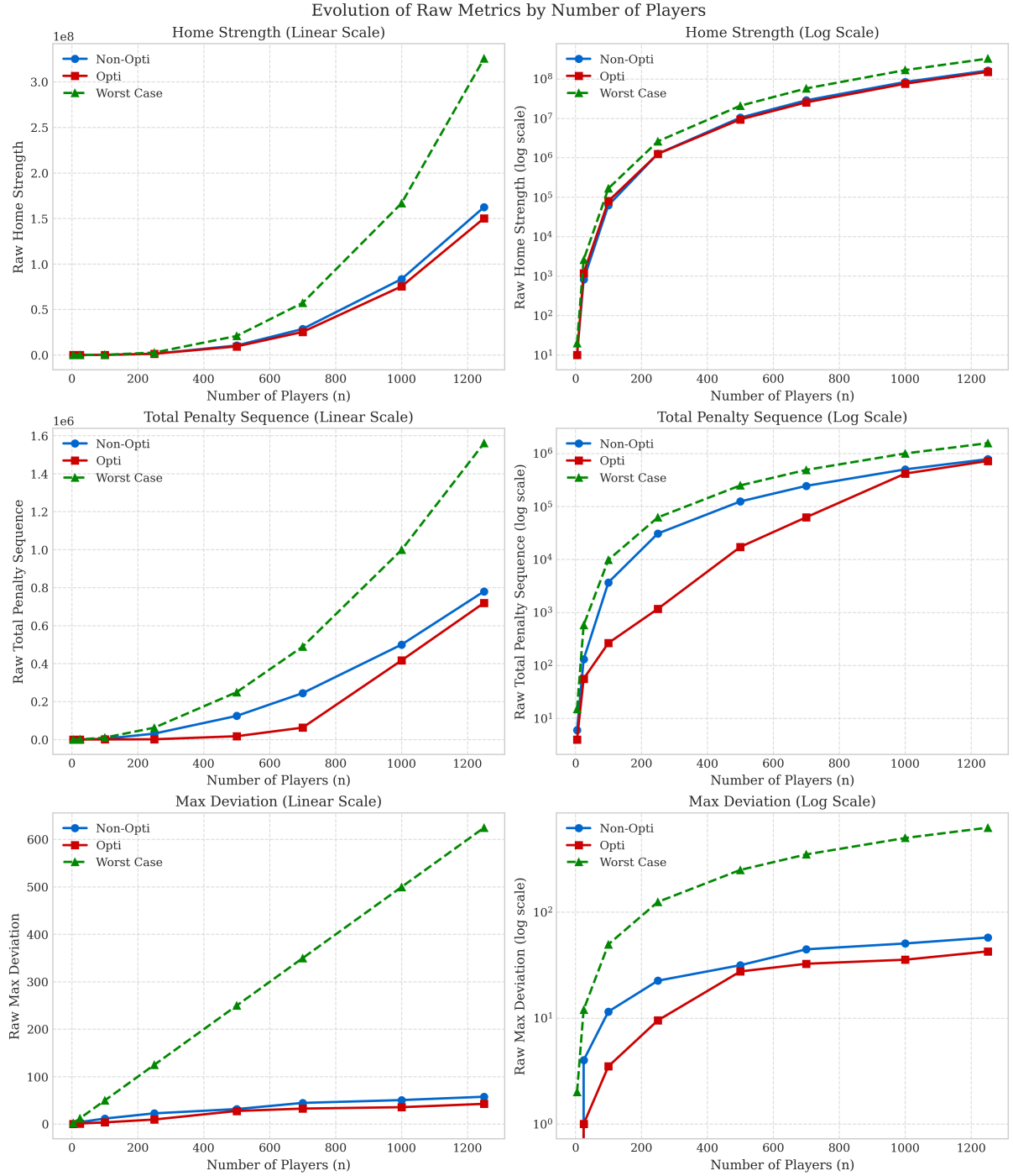
FIGURE 2 – Évolution des valeurs brutes de HomeStrength (HS), Penalty Sequence (PS) et Max Deviation (MD) en fonction de n pour les versions Non-Opti (bleu) et Opti (rouge) du Recuit Simulé, comparées au pire cas théorique (vert). Chaque point correspond à la meilleure solution trouvée en 60 s.
