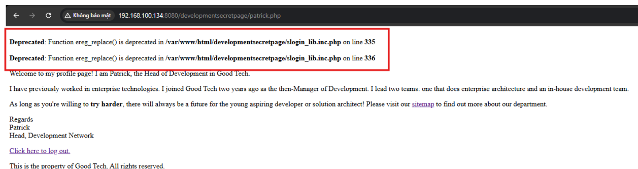
Hình 28: Trả lại trang web ban đầu nhưng lại gồm 2 dòng báo lỗi của php. Từ file slogin_lib.inc.php
