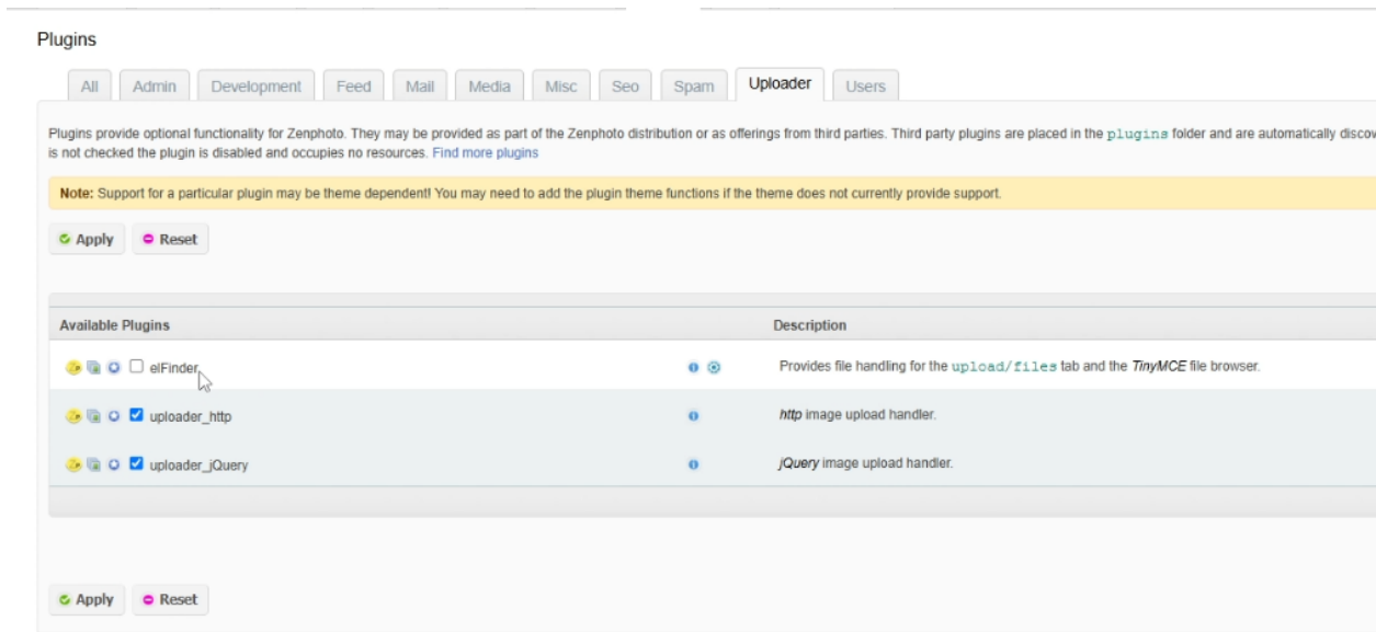
Hình 16: Ta tìm thấy 1 plugin Upload chưa được active trong hệ thống
