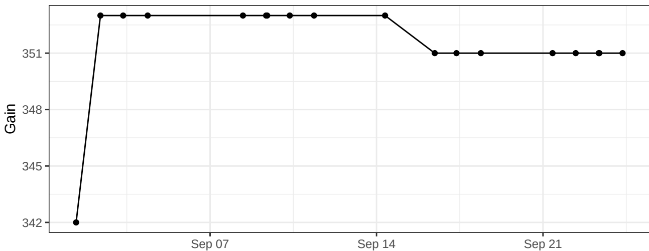
BUV615-A_Gain
